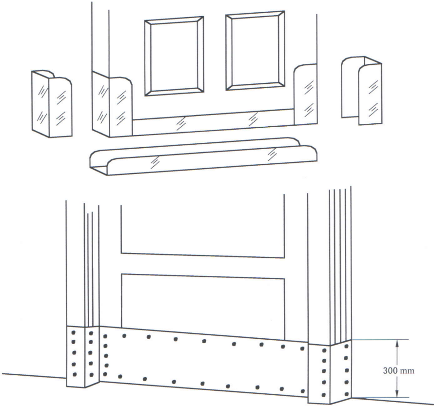
图 B.1 门及门框的镶包方式
